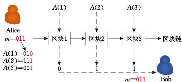
图 7 BLOCCE [95] 执行流程
