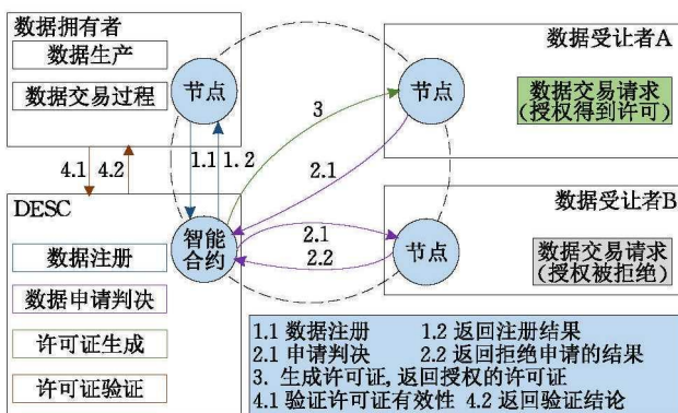
图 8 DECS [101] 工作流程
