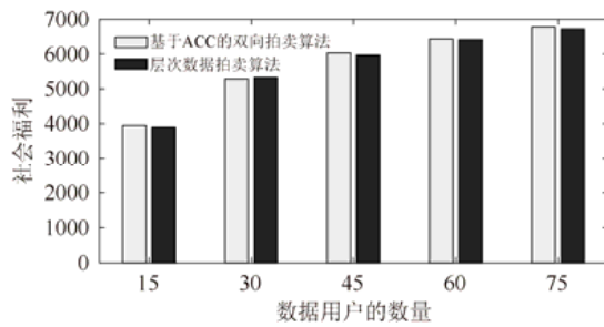
Fig.10 Average maximum social welfare in hierarchical data auction and double auction algorithms 图 10 层次数据拍卖算法和基于 ACC 的双向拍卖算法的最大社会福利
