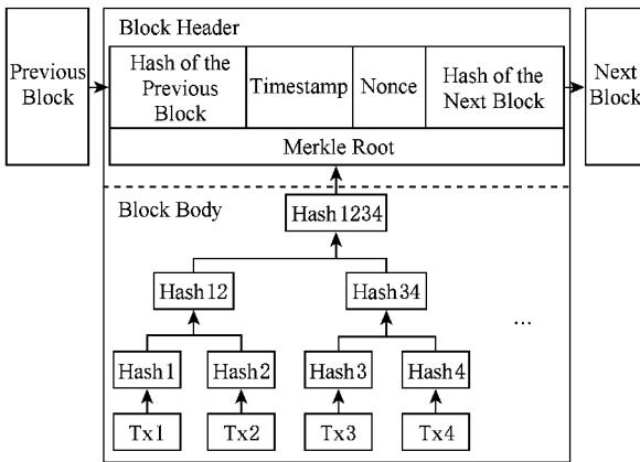
Fig. 1 Structure of block 图 1 区块结构
